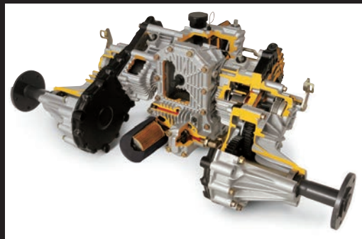
Originální převodovka Kubota
